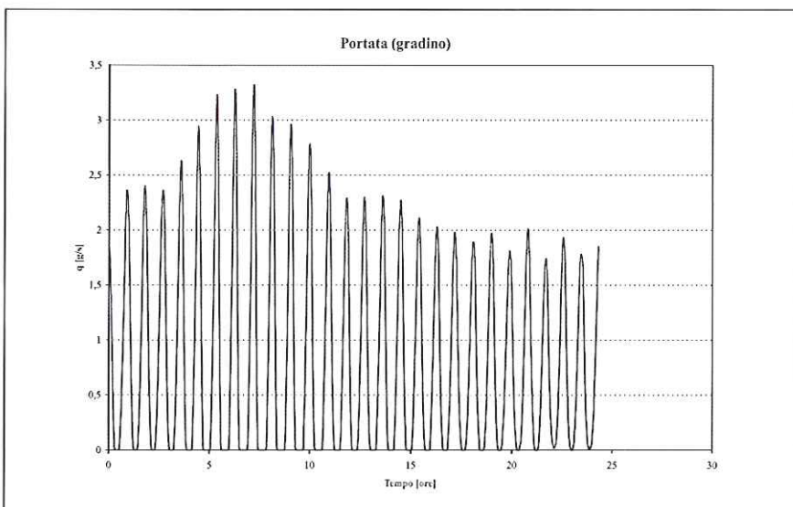
Fig. n. 2: Grafico della portata di una valvola termostatica ad inerzia non sufficientemente bassa, che entra in oscillazione al tentativo di conferirle elevata autorità.
